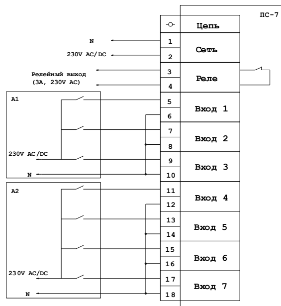
Рис. 2 — Схема подключения панели сигнальной.
