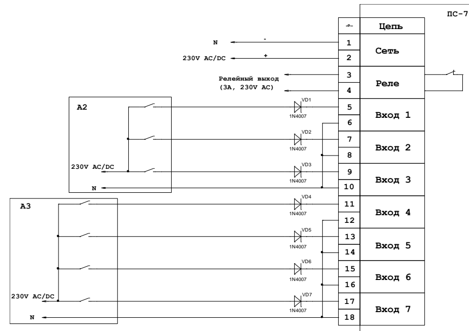
Рис. 3 — Схема подключения панели сигнальной в условиях помех.
