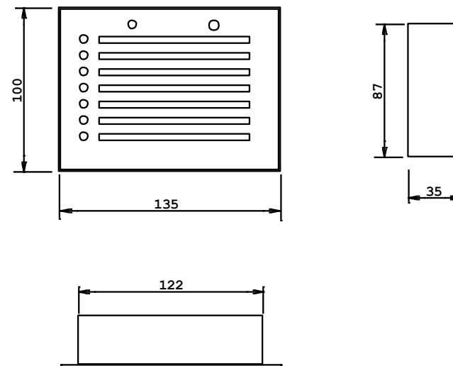
Рис. 1 — Габаритные размеры ПС-7.У3.
