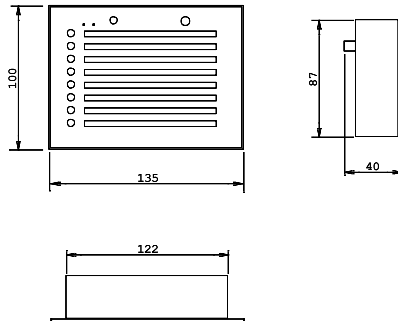
Рис. 1 — Габаритные размеры ПС-8М.У3. (рекомендуемый размер окна в щите 124x89 мм)
