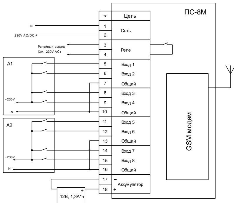
Рис. 2 — Схема подключения панели сигнальной
